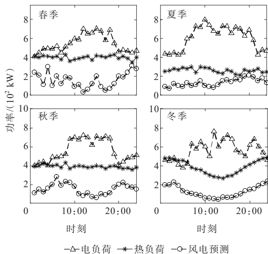
图2 典型日风电机组预测曲线和电、热负荷曲线
