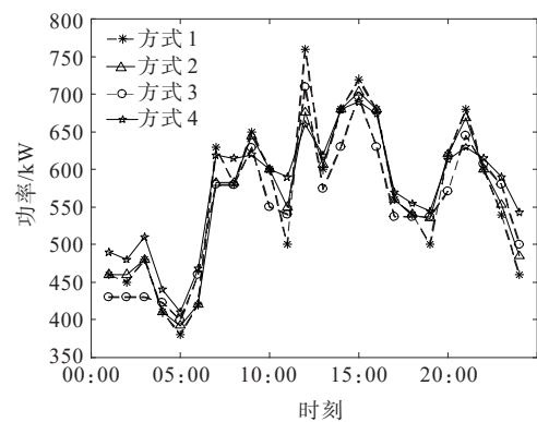
图3 4种运行方式下电负荷曲线
