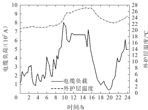
图 10 线路实时负载与外护层温度
