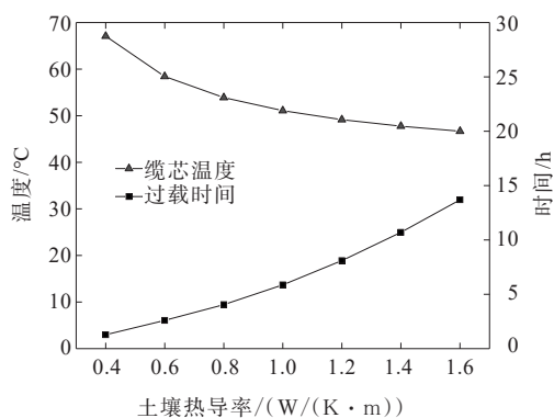
图5 过载时间与土壤热导率关系
