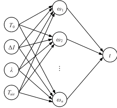
图8 BP神经网络模型
