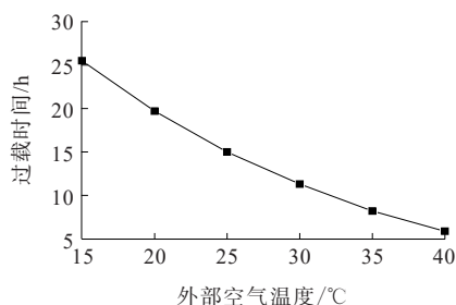
图7 过载时间与外部空气温度关系
