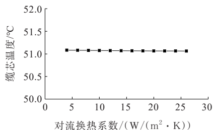
图6 缆芯温度与对流换热系数关系
