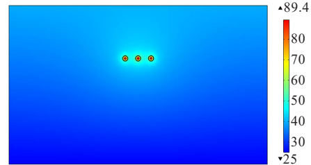
(b) 缆芯温度接近 90^\circ\text{C} 时暂态温度场
