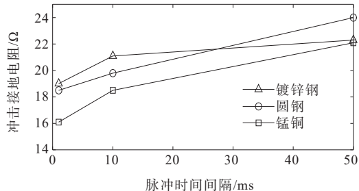
图5 一字型接地体的冲击接地电阻
