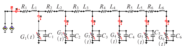
图7 连续冲击下水平接地体仿真模型
