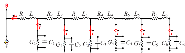
图6 水平接地体ATPDraw仿真模型
