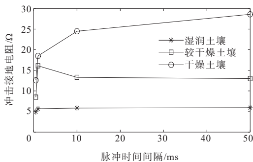
图3 不同含水量土壤中水平接地体的冲击接地电阻
