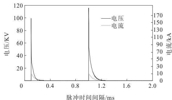
图8 连续冲击下水平接地体仿真波形
