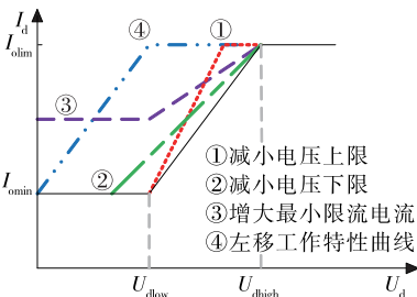
图 6 优化 VDCOL 工作特性曲线
