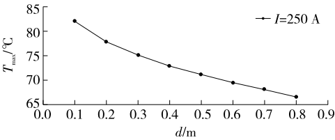
图 13 双根电缆缆芯间距对电缆运行时最大温度 T_{\max} 的影响
