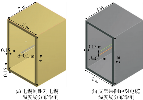
图 2 双根电缆铺设几何模型
