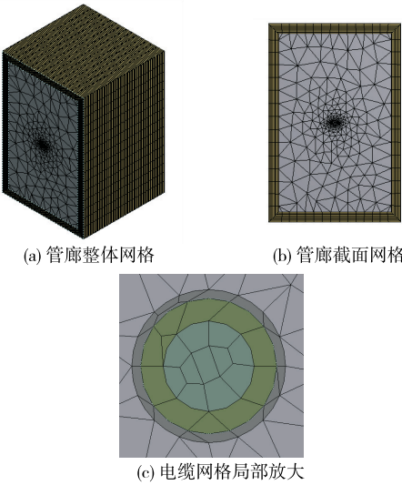
图 3 模型网格划分
