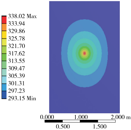
图 4 单根电缆温度场分布云
