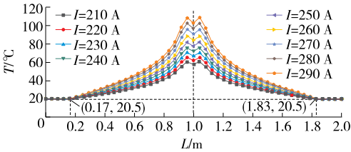
图 10 电流对电缆温度场分布的影响
