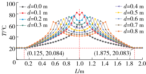
图 12 双根电缆缆芯间距对温度场分布的影响
