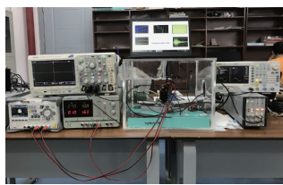
(a) 测试系统实物
