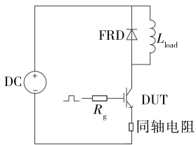
(b) 电路原理示意
