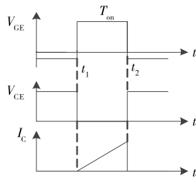
图 4 脉冲测试时序
