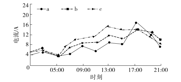
图 3 降损前配电网三相电流情况
