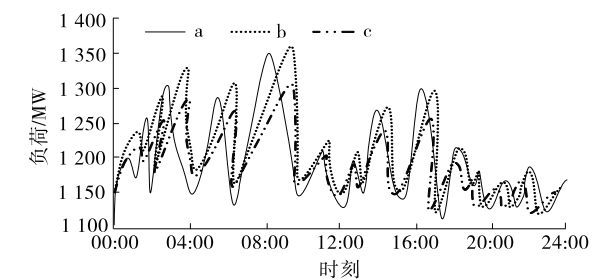
图 2 三相不平衡配电网的负荷情况
