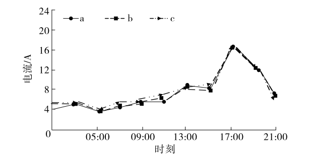
图 4 降损后配电网三相电流情况
