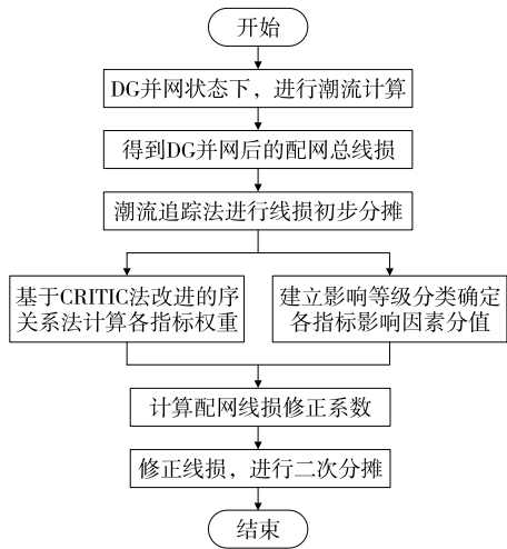
图 7 兼顾 DG 影响等级划分及权重特性的线损分摊方法流程
