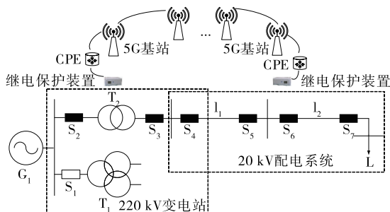
图 7 仿真模型
