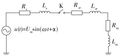
图 1 变压器空载合闸等效电路
