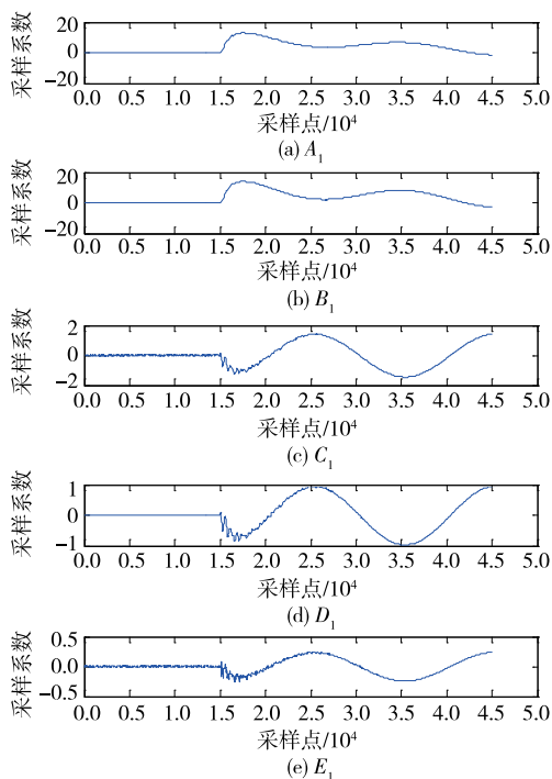
图 4 各监测点的小波包低频重构系数
