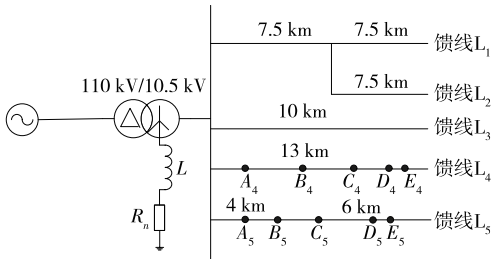
图 6 仿真模型 Figure 6 Simulation model
