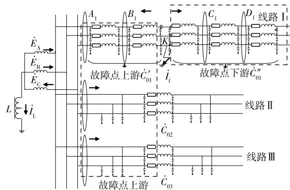
图 1 配电网单相接地故障零模网络等效电路
