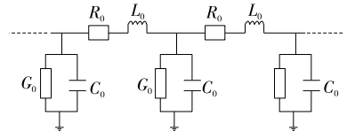
图 1 有损长线模型
