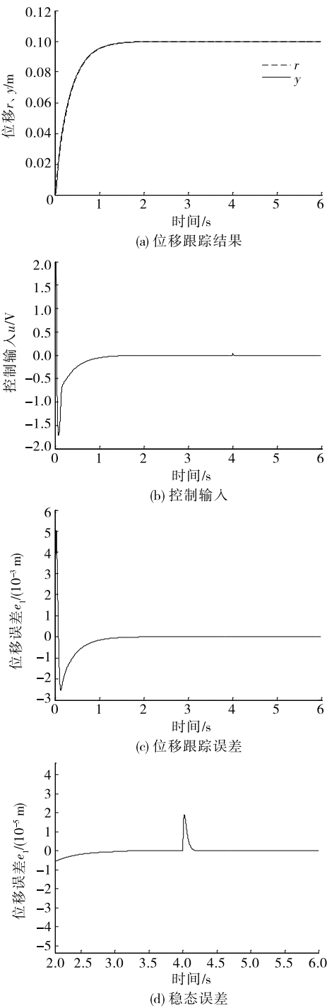
图 3 自耦 PD 控制结果
