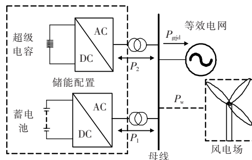
图 1 风储联合发电系统的结构
