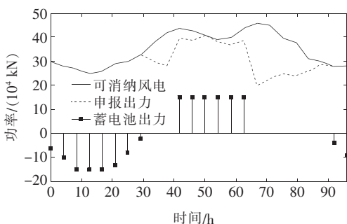
图 3 蓄电池配置效果示意
