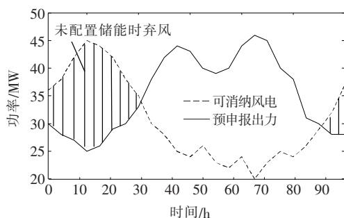
图 2 某月典型日的风电示意
