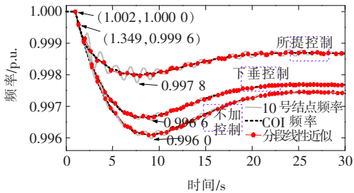
(a) 15 号节点吸收功率突增 3.0 p.u.时的系统频率变化过程
