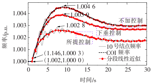
(b) 4 号节点吸收功率突降 3.0 p.u.时的系统频率变化过程
