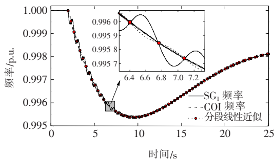
图 2 两机系统受扰后的频率响应
