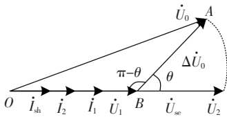
图 5 PEVR 稳态时电压电流相量
