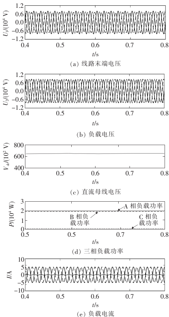
图 10 三相负载不平衡时电压补偿波形
