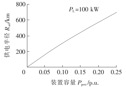
图 6 装置容量和供电半径的关系曲线
