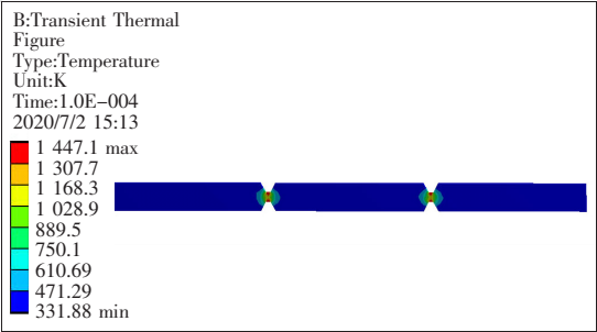
图 3 雷电流幅值为 20 kA 时熔体在 t=100\ \mu\text{s} 时温度分布
