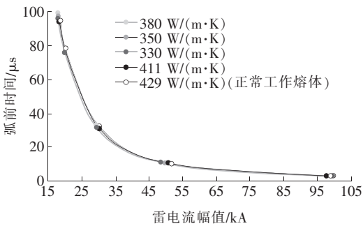
图 4 不同热传导系数下熔断器雷电流幅值—弧前时间对比
