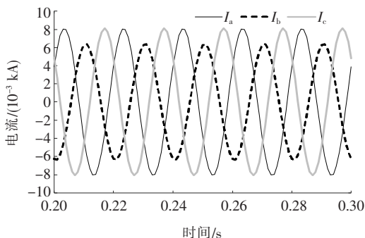
图 14 首次换相后三相电流
