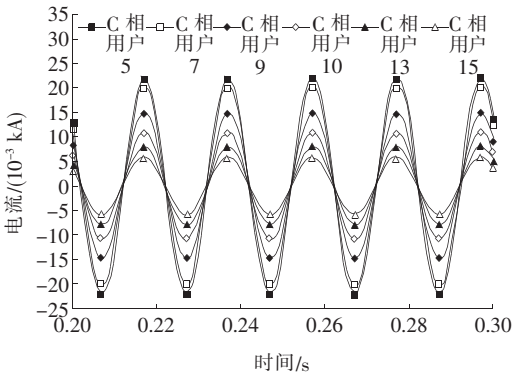
图 9 换相前 C 相各换相单元电流波形 Figure 9 Currents of phase C before commutation
