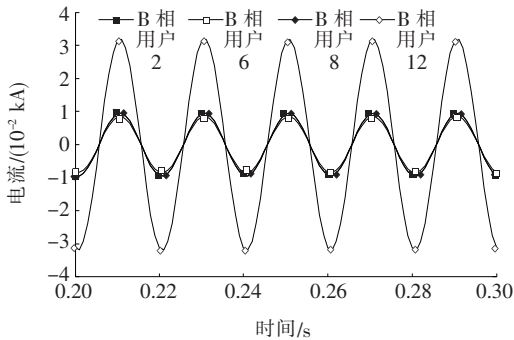
图 8 换相前 B 相各换相单元电流波形 Figure 8 Currents of phase B before commutation
