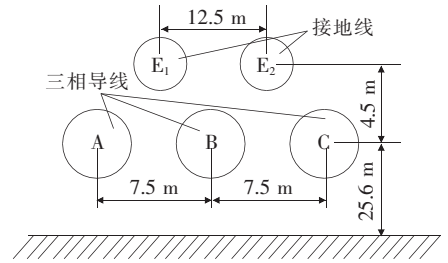
图4 架空线排布
