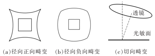
图4 径向和切向畸变产生原因示意
