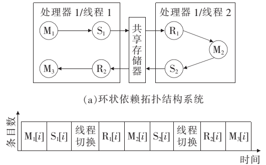
(b) 核内双条目缓存系统执行序列
