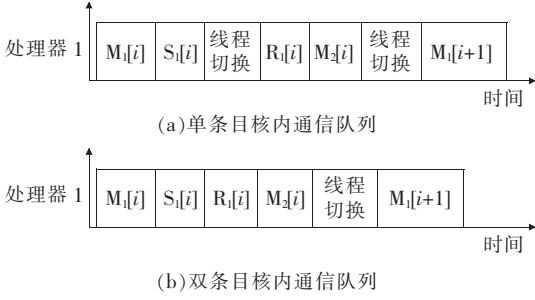
图 3 核内通信队列的执行序列
