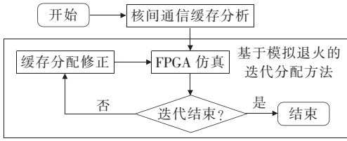
图 4 基于 FPGA 的核间通信队列分派
