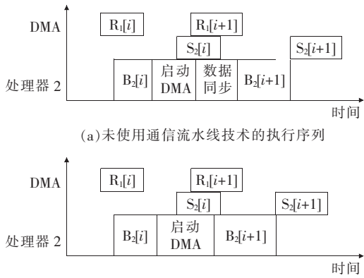
图 8 通信流水线的优势
