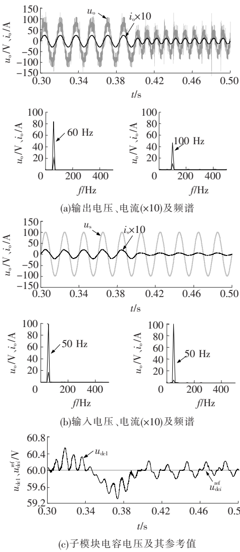
图 6 采用所提 MPC 算法的动态响应波形
