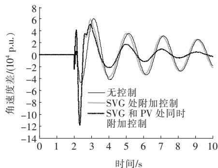
图 6 三相接地时同步发电机 1、3 角速度差
