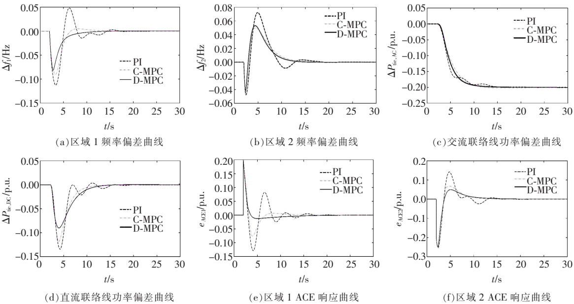
图 6 3 种方法的系统动态响应性能对比(案例 1)
