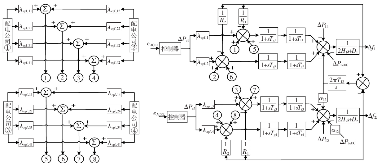
图 2 基于 DPM 的负荷频率控制模型
