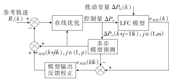
图 3 模型预测控制原理
