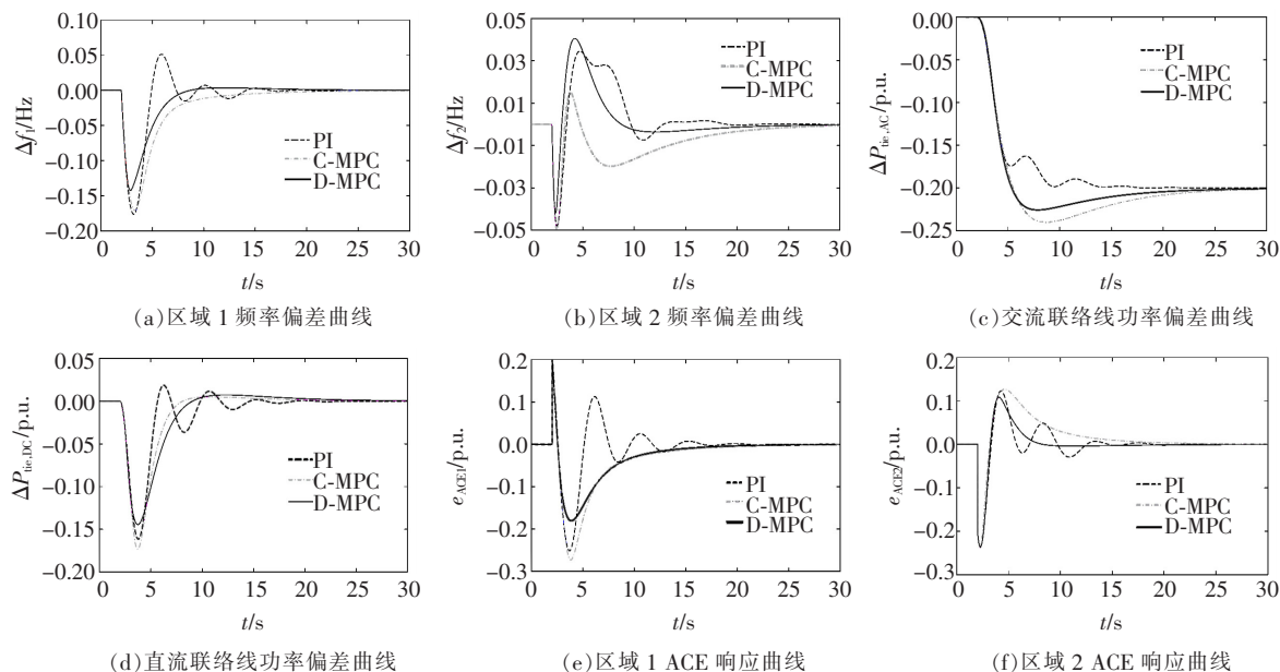
图 7 3 种方法的系统动态响应性能对比(案例 2)
