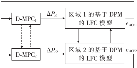
图 5 分布式模型预测控制结构
