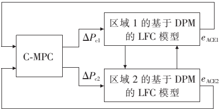
图 4 集中式模型预测控制结构
