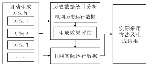
图 1 算法特征
