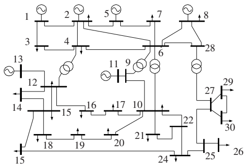
图 4 IEEE 30 节点模型
