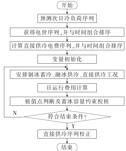
图2 趋优控制方法流程
