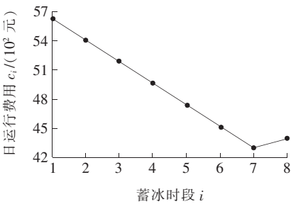
图 3 日运行费用的变化情况
