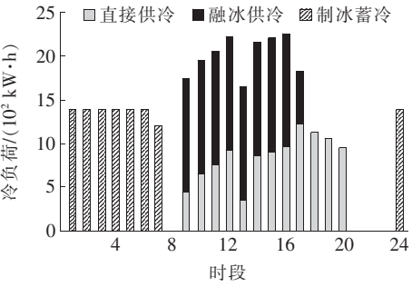
图 5 融冰优先控制策略下的冷量分配
