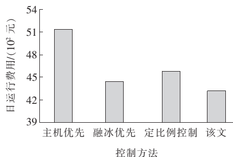
图 7 4 种控制方法的日运行费用比较
