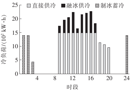
图 4 主机优先控制策略下的冷量分配
