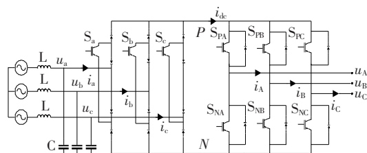
图 1 USMC 拓扑结构
