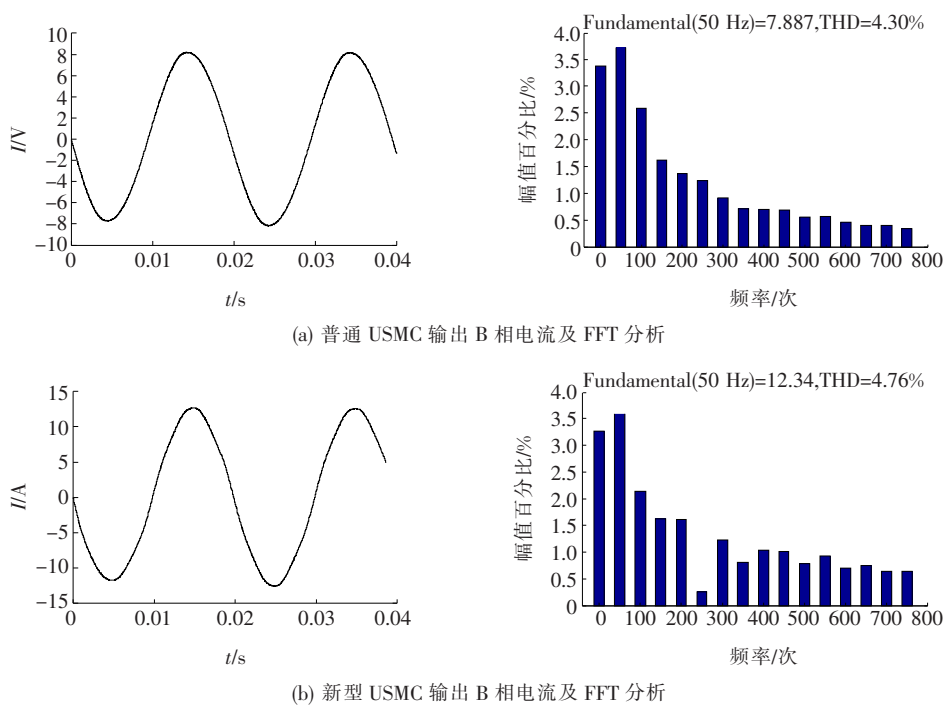
图 9 普通与新型 USMC 输出相电流及 FFT 分析
