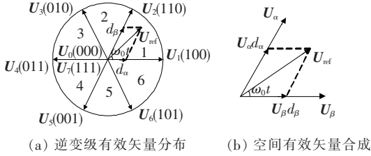
图 4 USMC 逆变级空间有效矢量分布及合成调制
