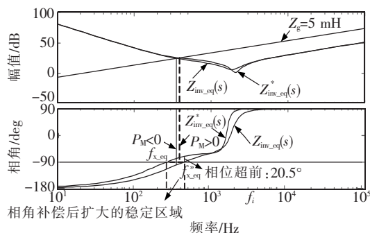
图 6 Z_{\text{inv\_eq}}(s) 和 Z_{\text{inv\_eq}}^*(s) 的波特特性
