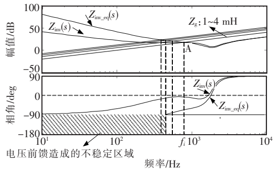
图4 Z_{\text{inv\_eq}}(s) 和 Z_{\text{inv}}(s) 的波特特性
