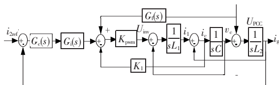
图 5 加入相位超前补偿后的双环电流控制结构
