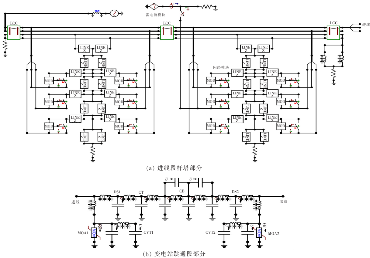
图 4 雷电过电压计算模型 Figure 4 Lightning overvoltage calculation model
