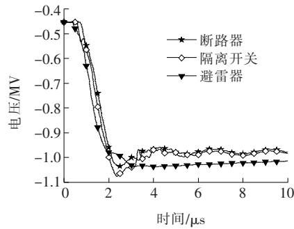
图 6 绕击 #1 塔时设备侵入波过电压波形
