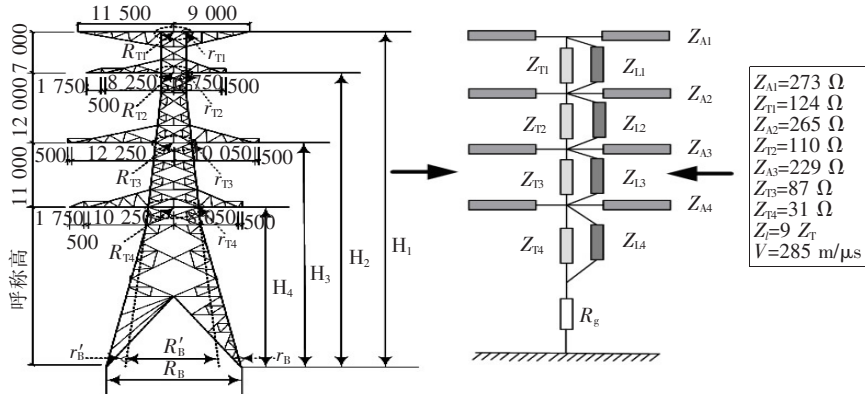
图2 杆塔多波阻抗模型
