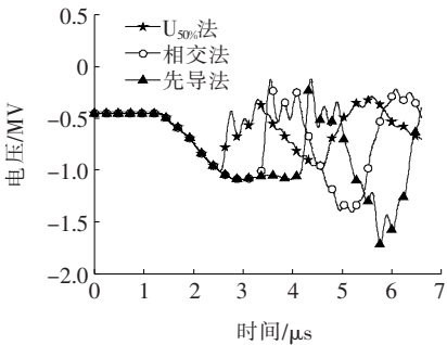
图 10 不同闪络模型下断路器过电压波形
