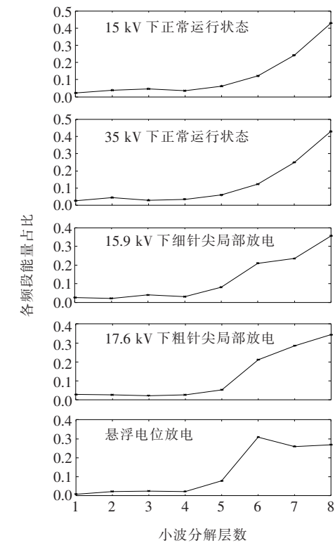
图 14 不同工况下各频段信号能量占比
