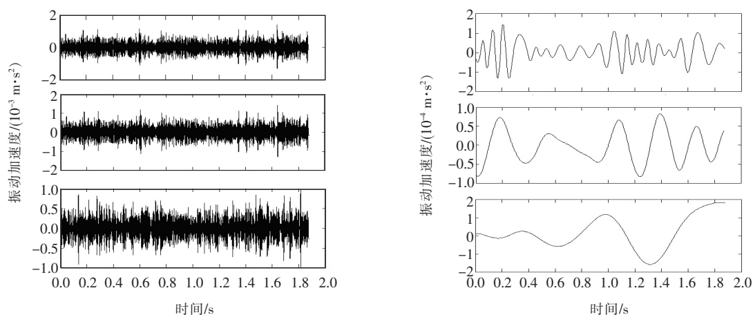
图8 正常运行条件下的 MEEMD 分解
