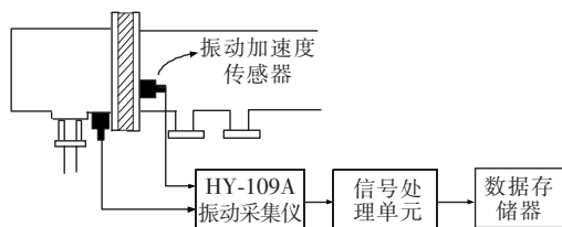
图 2 GIS 振动信号采集系统
