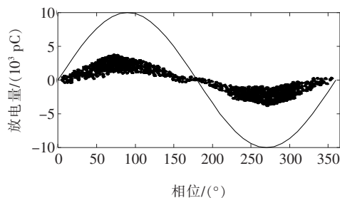
图 3 悬浮金属颗粒物放电相位特征
