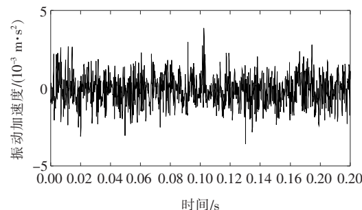
图 7 GIS 局部放电的振动信号
