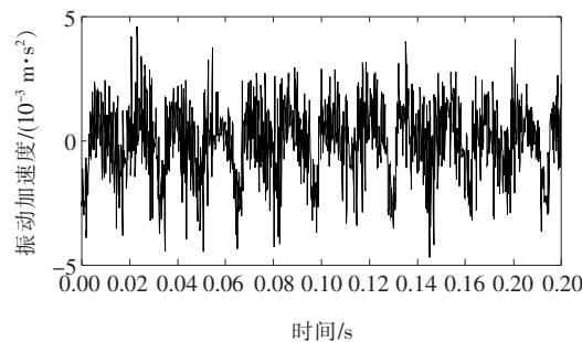
图 6 GIS 绝缘子松动时振动信号
