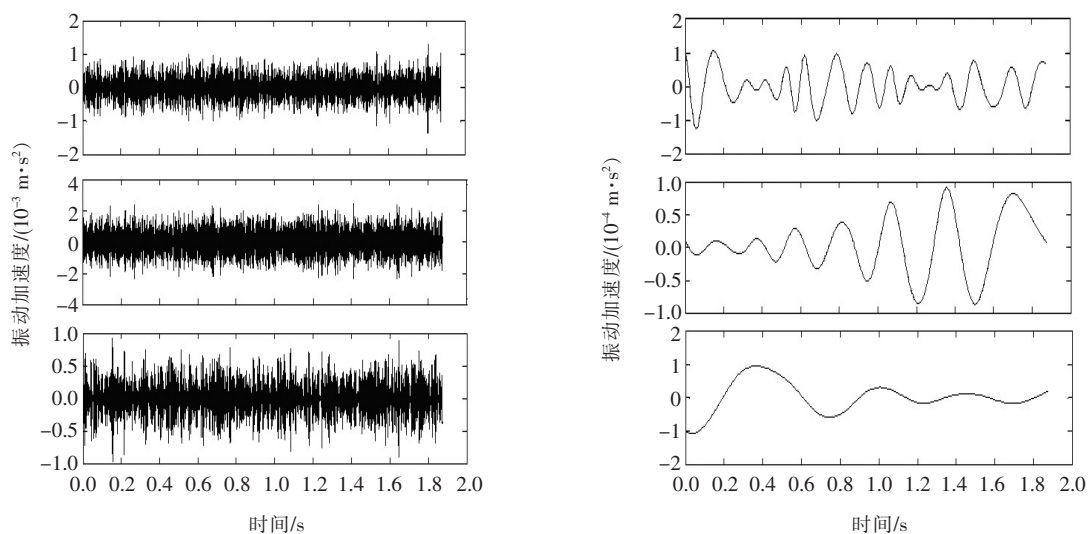
图10 局部放电下的 MEEMD 分解
