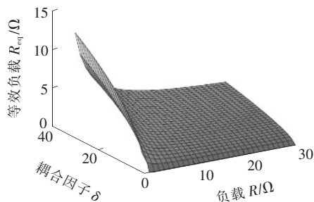
图 4 负载 R 、耦合因子 \delta 与等效负载 R_{eq} 的关系曲线
