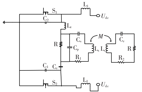
图 10 改进的电路模型 Figure 10 Improved circuit model
