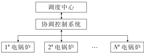
图 1 蓄热消纳系统结构
