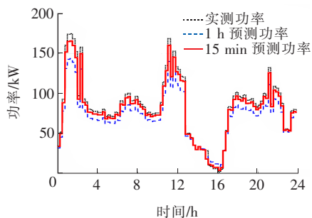
图 3 某风场某风电场日内风功率曲线
