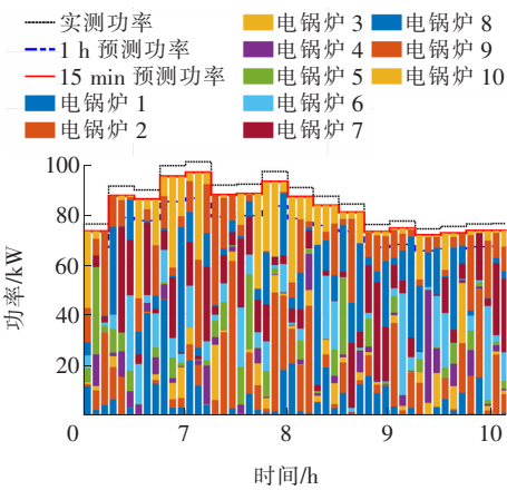
图 5 8:00 时的消纳功率优化结果
