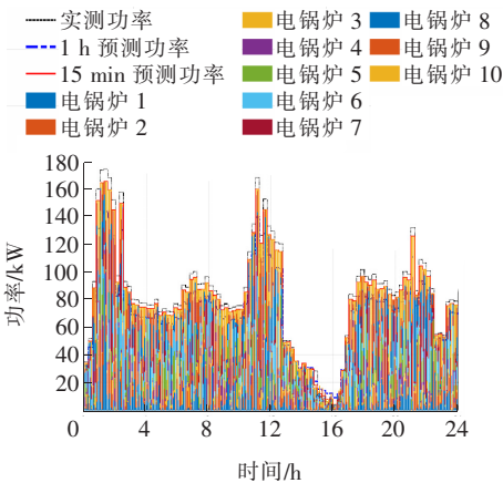
图 4 蓄热电锅炉消纳功率优化结果
