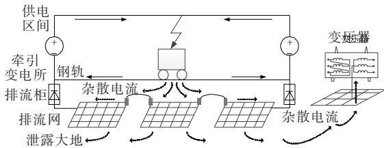
图 1 杂散电流引起变压器直流偏磁示意
