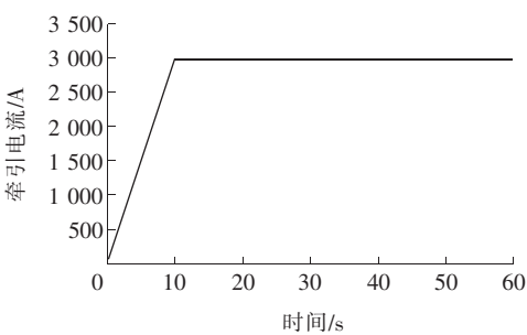
图 5 地铁牵引电流随时间变化曲线
