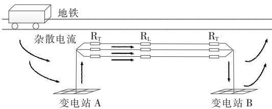
图 2 杂散电流流通回路示意
