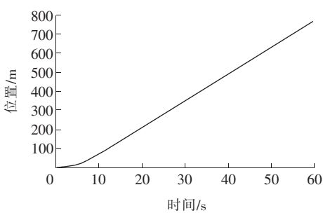
图 6 地铁位置随时间变化曲线
