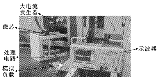
图 7 实验平台
