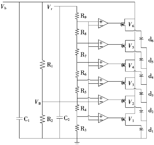
图 5 锂电池电量监测电路
