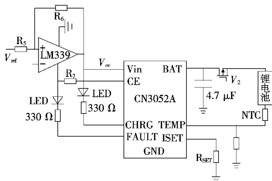
图 4 充电电路
