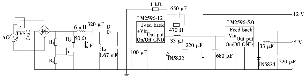
图 3 双路输出电路
