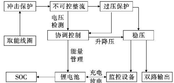
图 2 电源结构
