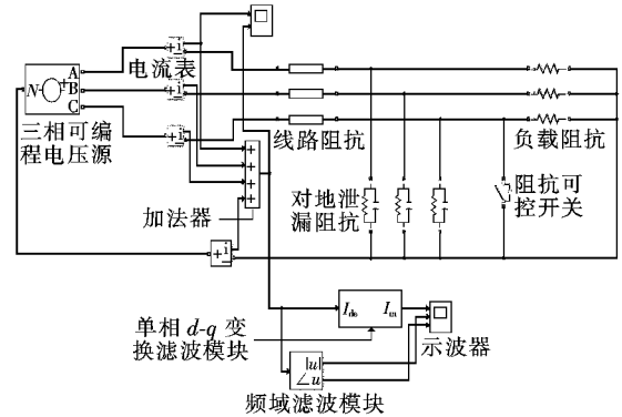
图 4 仿真电路
