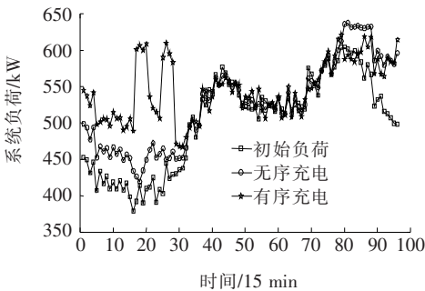
图 8 EV 有序充电与无序充电对比
