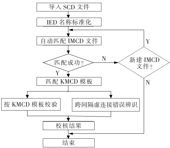
图 1 虚回路自动校验流程
