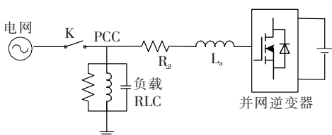
图 1 孤岛运行结构
