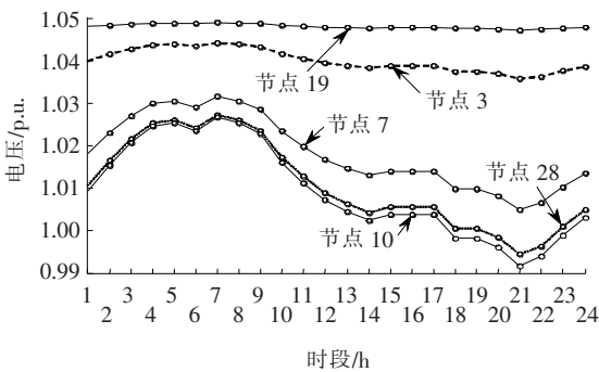
图 8 ADN 中 DG 接入节点电压幅值随机模糊期望值 Figure 8 DG bus magnitude random-fuzzy expectation in ADN
