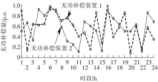
(c)无功补偿量
