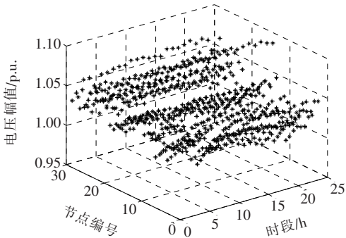
(b)日前最大满意度决策下的 TS 电压幅值随机模糊期望值
