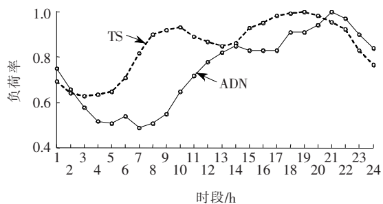
图 3 TS 日负荷
