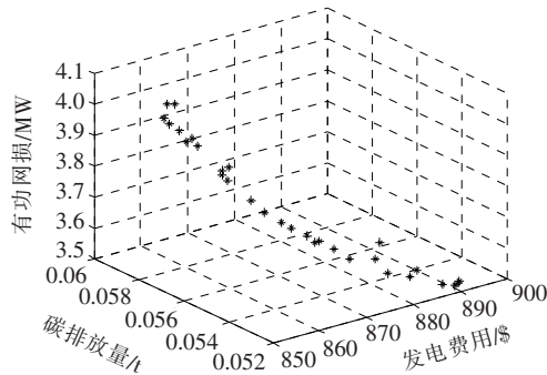
图 4 14 时段 Pareto 前沿图
