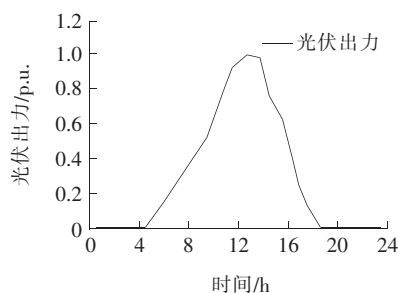
(b) 光伏曲线
