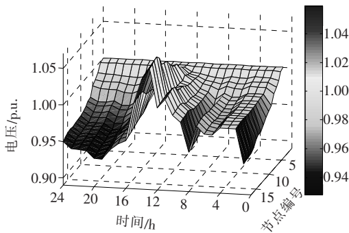
图 4 补偿后节点 1-18 的电压
