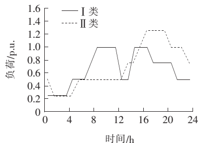
(a) 负荷曲线
