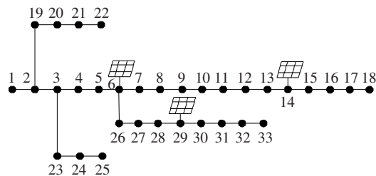
图 1 IEEE33 节点测试系统
