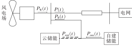
图1 风电场配置自建及云储能的系统架构
