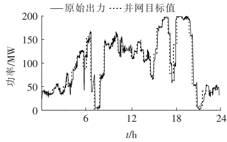
图 2 风电场原始出力曲线及并网期望曲线
