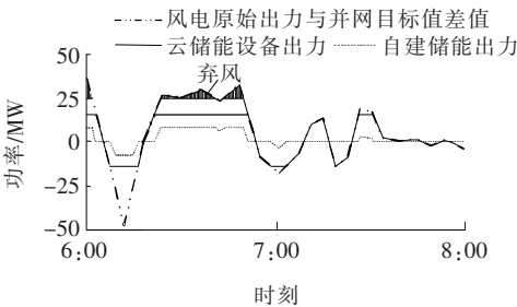
图 3 情景 1 部分时刻自建与云储能系统充放电功率
