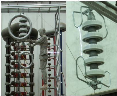
图 1 试验现场 Figure 1 Test site pictures
