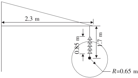
图 3 直线塔作业间隙
