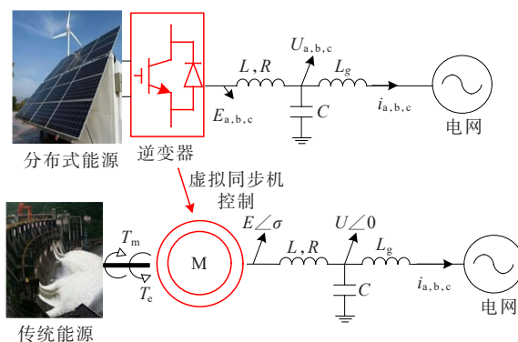
图1 同步发电机等效电路模型
