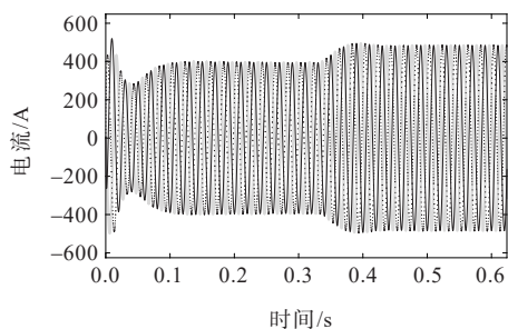
(b) 输出三相电流波形
