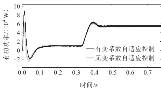
(a) 有功功率的输出波形
