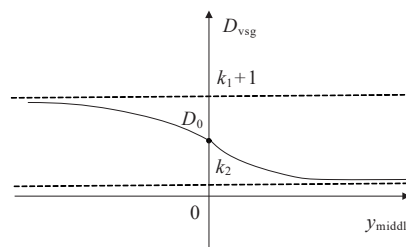
(b) 旋转阻尼与频率的关系曲线
