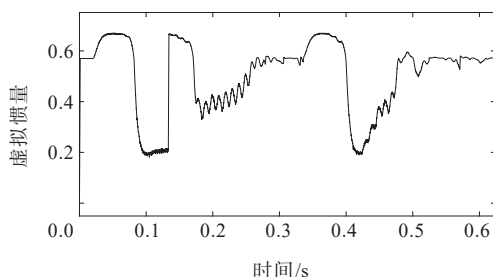
(b) 阻尼系数波形
