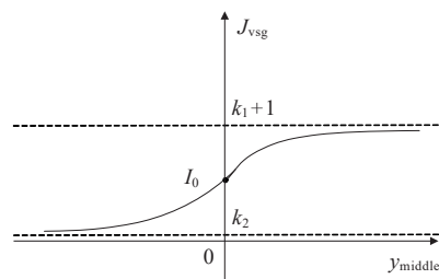
(a) 虚拟惯量与频率的关系曲线
