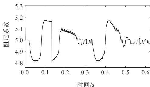
(a) 虚拟惯量波形
