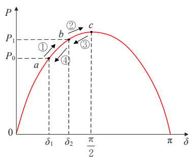
(a) 功角曲线
