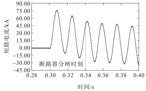
图 8 短路电流实际波形
