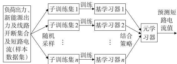
图 4 Bagging 集成学习结构
