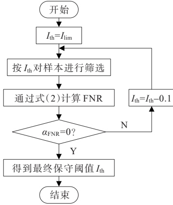
图2 保守阈值整定流程
