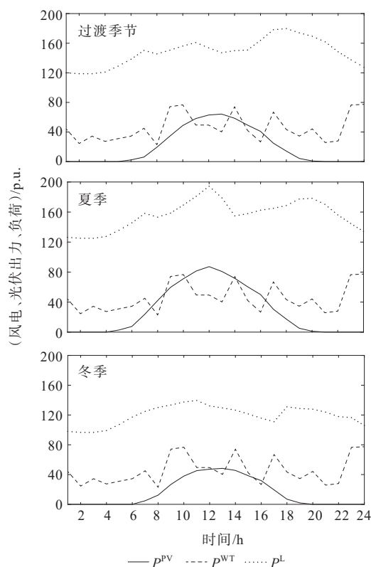
图3 过渡季节、夏季以及冬季典型日风电、光伏出力及负荷曲线
