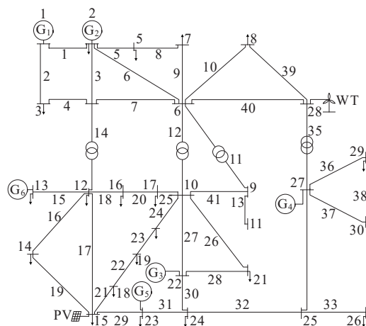
图2 算例系统示意
