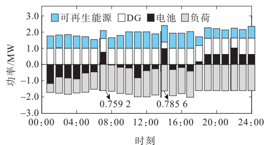
图10 方案1配电网功率分布情况
