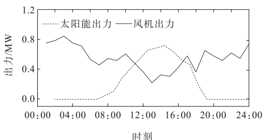
图7 可再生能源出力
