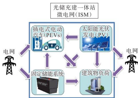
图1 ISM组成单元及其运行模式
