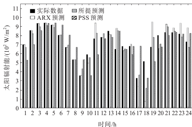
(a) 不同方法下太阳辐射预测对比
