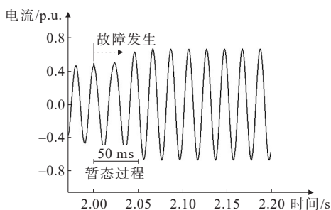
图8 逆变型电源故障输出
