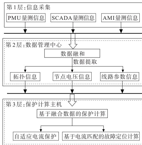
图 5 保护计算系统
