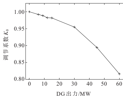
图10 不同出力下 K_0 变化趋势
