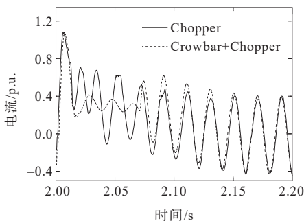
(b) Chopper电路投运
