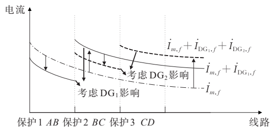
图 4 故障电流变化情况
