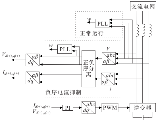
图 1 LVRT 控制策略
