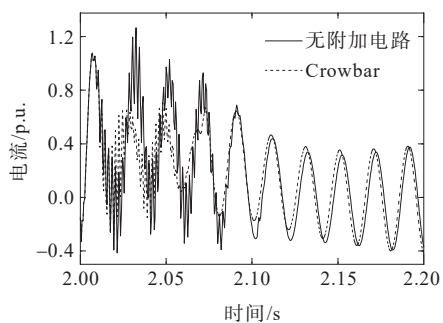
(a) 有、无附加电路投入
