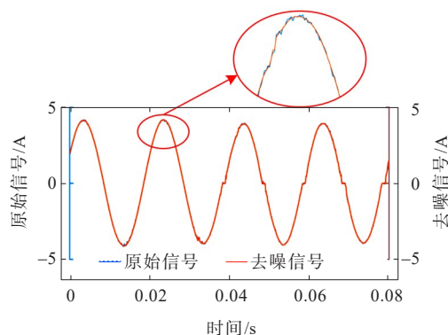
图6 信号去噪前、后波形对比
