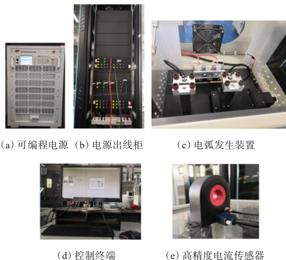
图5 实验原理与装置实物
