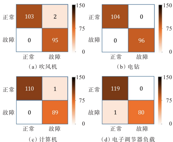
图10 故障临界区测试结果混淆矩阵
