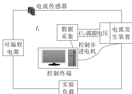
图4 实验平台接线原理
