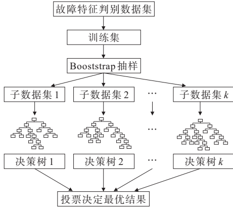
图2 随机森林算法结构原理
