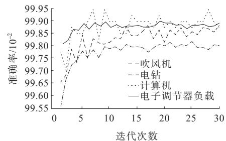
图9 交叉验证曲线
