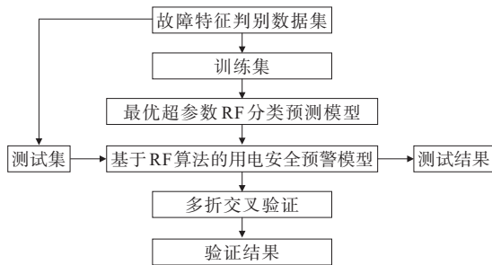
图8 用电安全隐患预警模型构建流程
