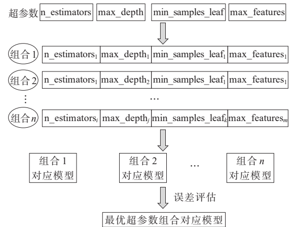
图3 模型超参数优化原理示意
